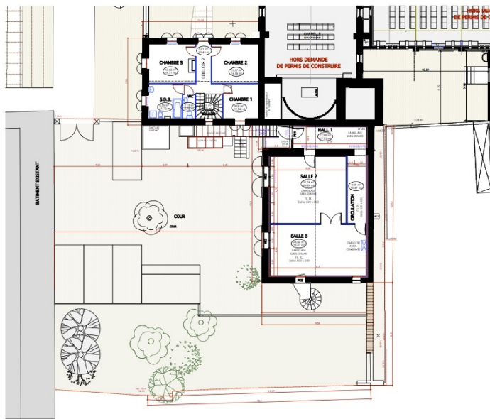
PLAN PROJET DE L'ÉTAGE
